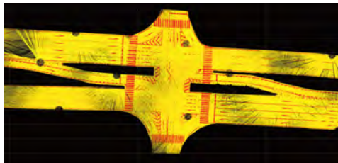
3次元点群ノイズ処理
