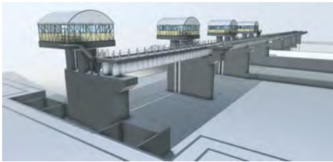
BIM/CIMモデル作成
