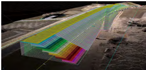
転圧・敷均しデータ作成
