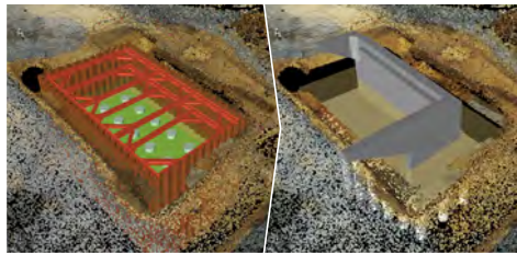
施工ステップ作成
